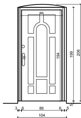
STRONA ZEWNĘTRZNA
