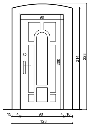
STRONA WEWNĘTRZNA
