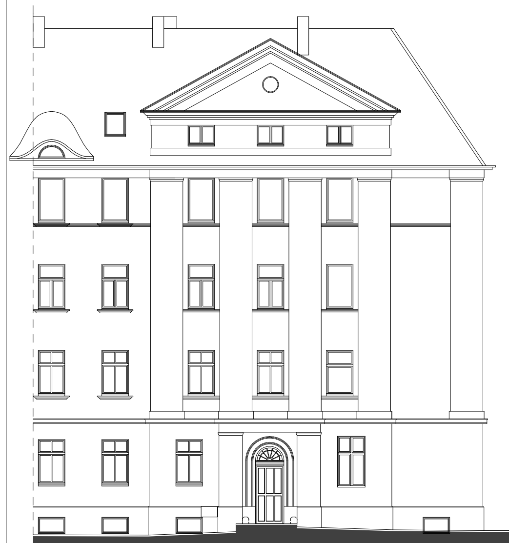
ELEWACJA UL. A. MICKIEWICZA 22
