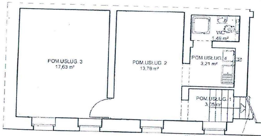
LOKAL UŻYTKOWY NR 1U Pu = 39,15 m 2
