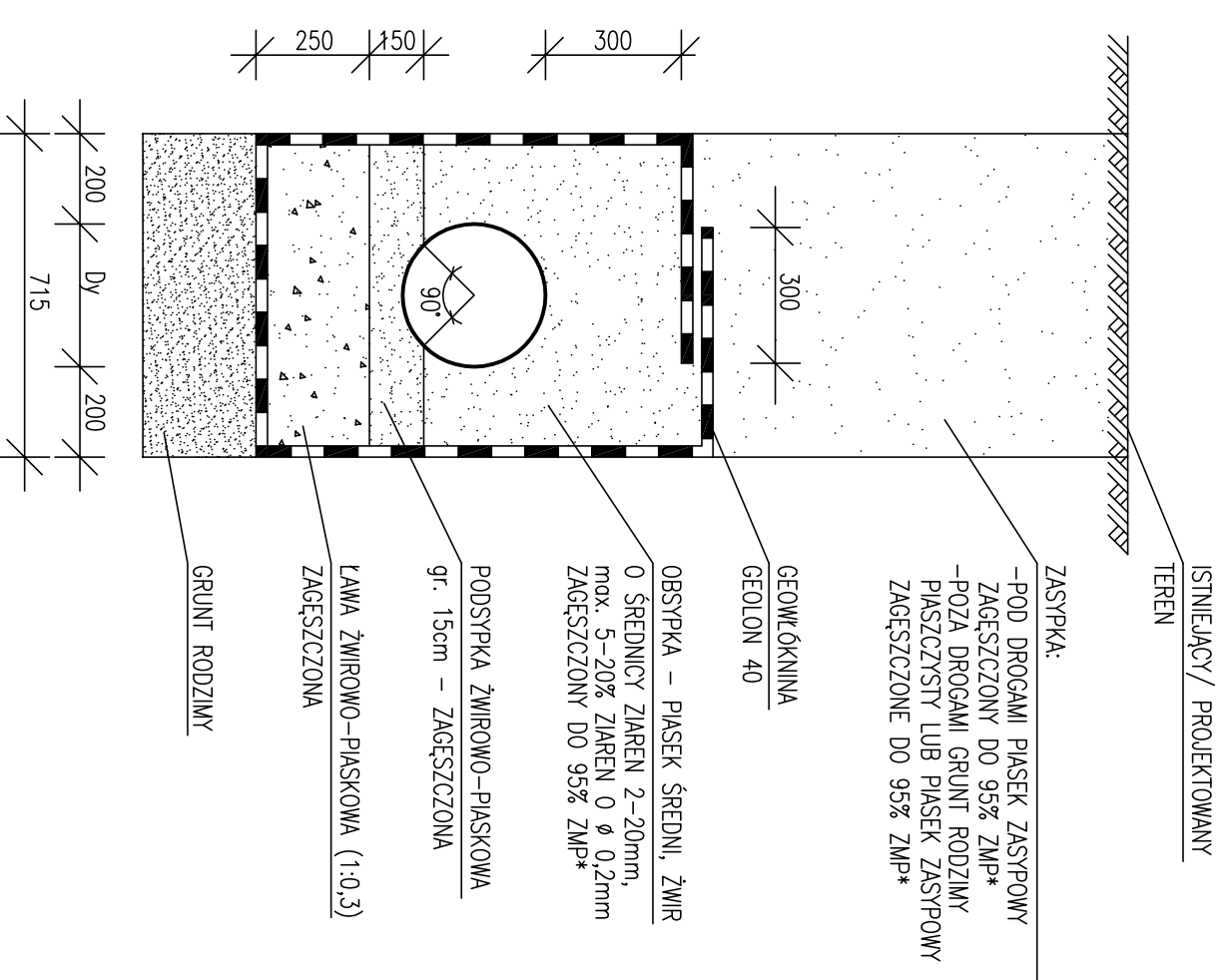
POSADOWIENIE TYP C
