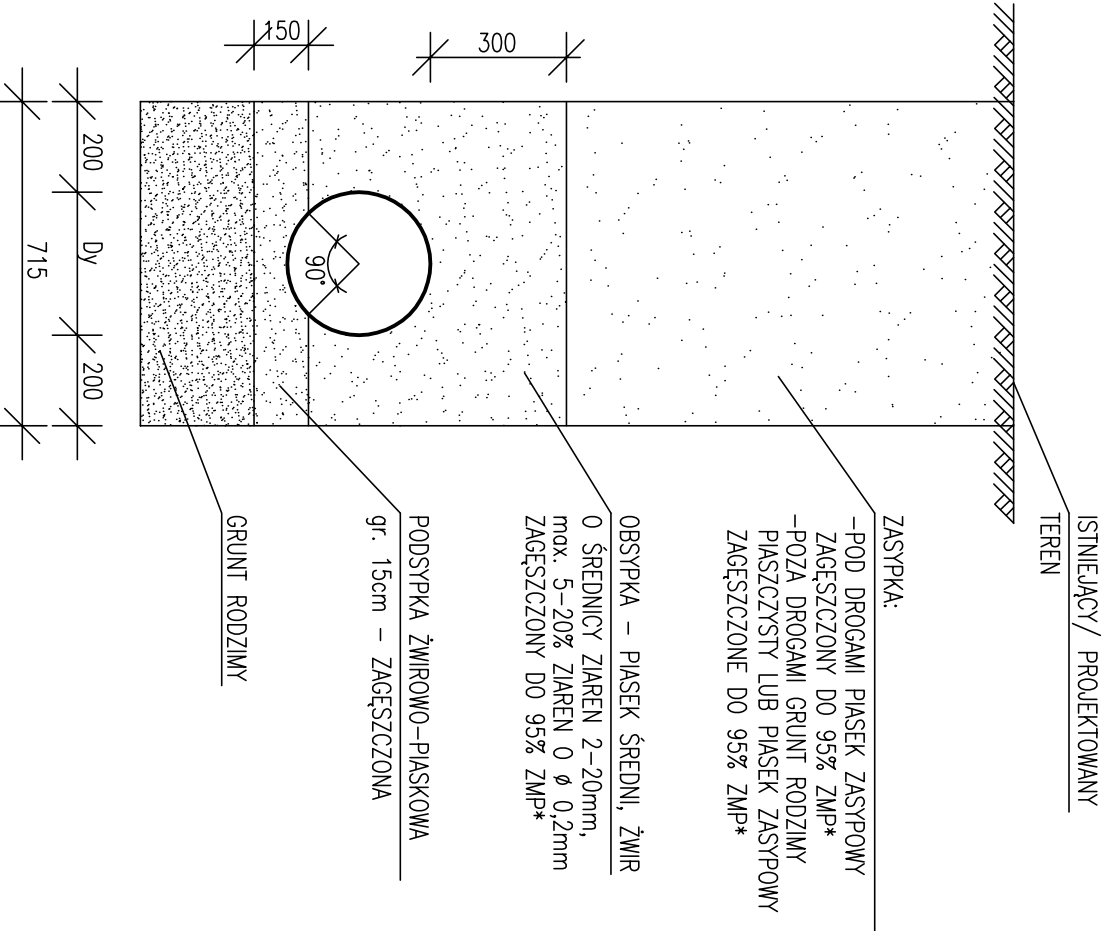
POSADOWIENIE TYP A
