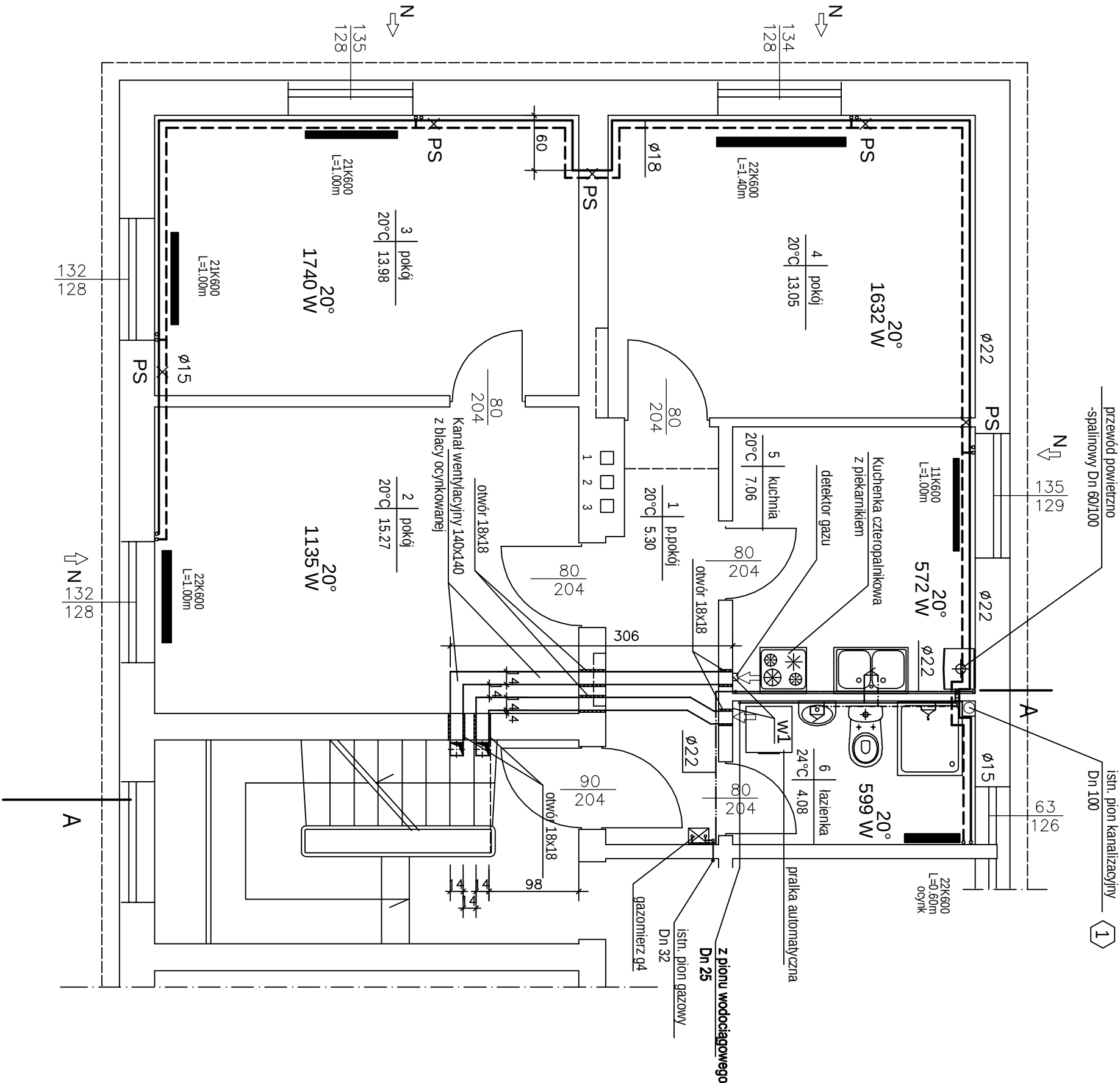
RZUT MIESZKANIA
